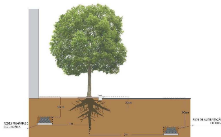
Figura 21- Espaçamento entre raízes e serviços públicos subterrâneos. Fonte: Architectus
